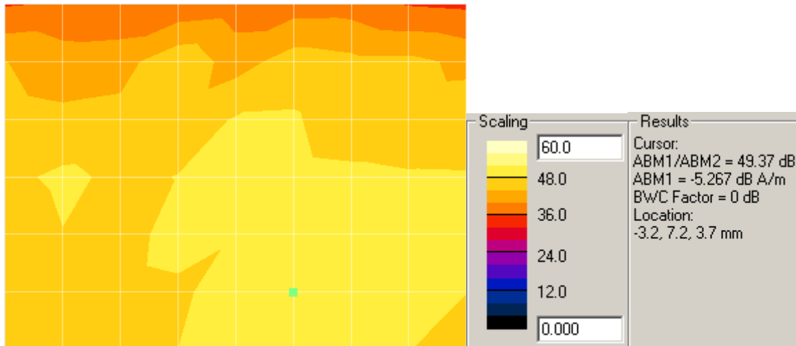
Radial2 – SNR
