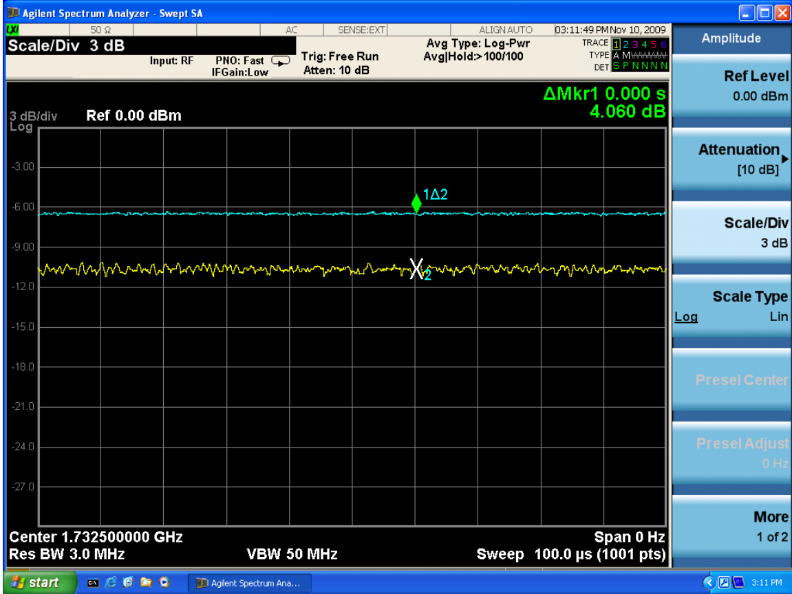
1700 EV-DO PAR Plot
