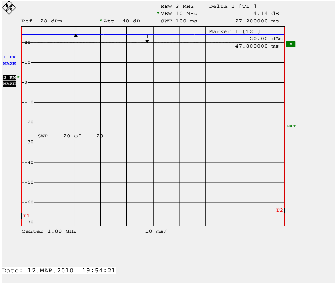
CDMA 1900 - PAR Plot
