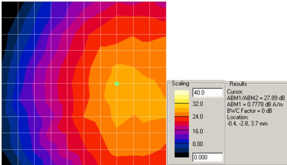
Axial – SNR
