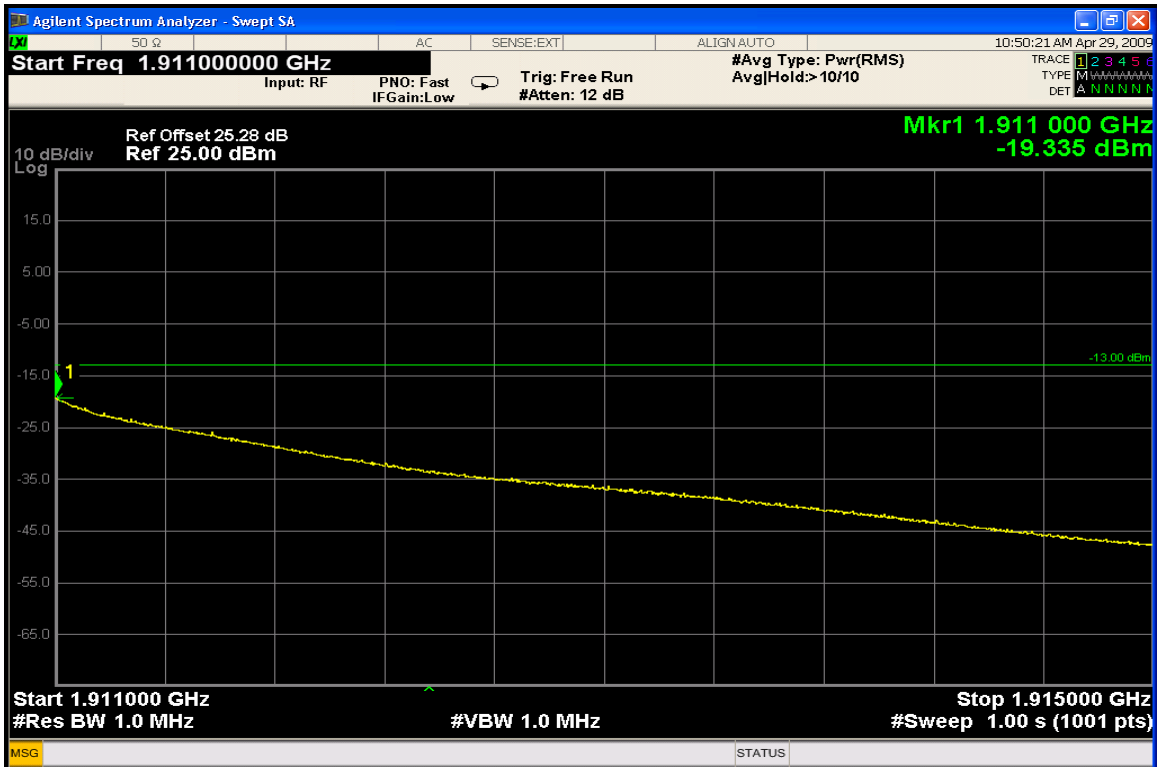
CDMA1900 Ch.1175 Upper Band Edge
