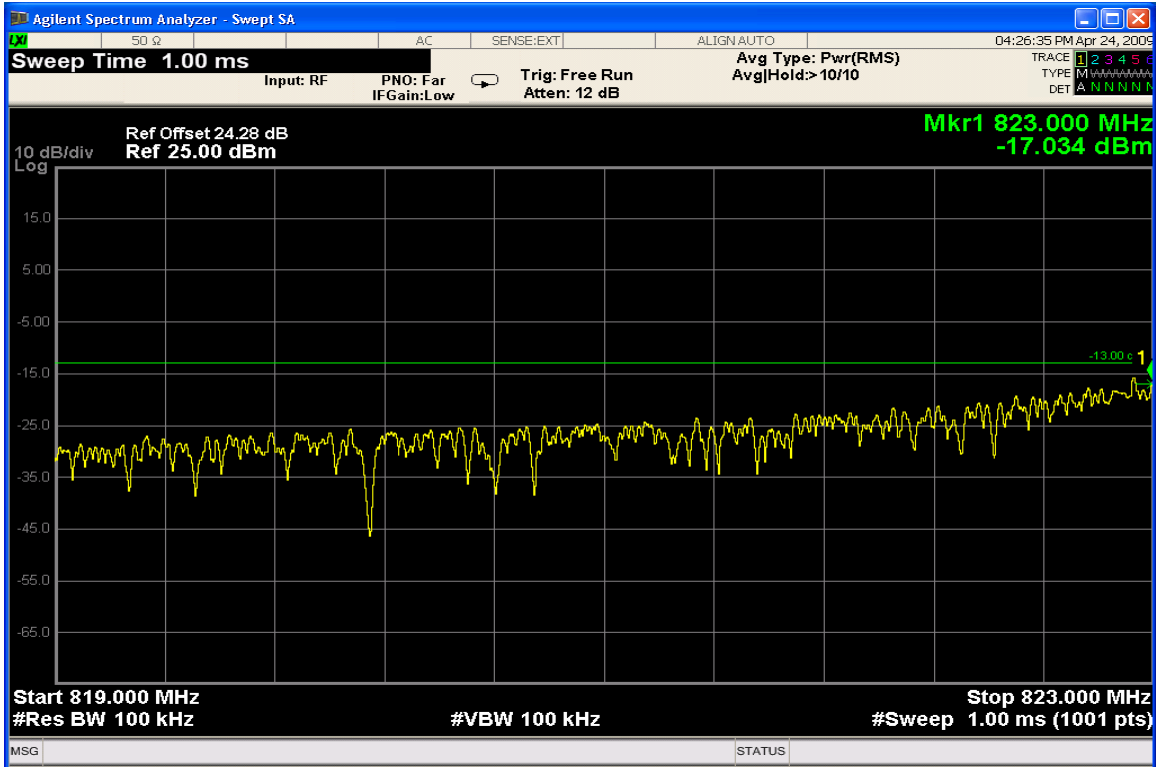
CDMA800 Ch.1013 Lower Band Edge
