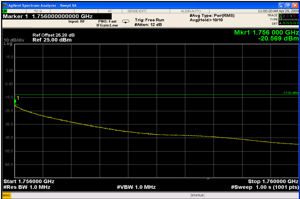
CDMA1700 Ch.875 Upper Band Edge
