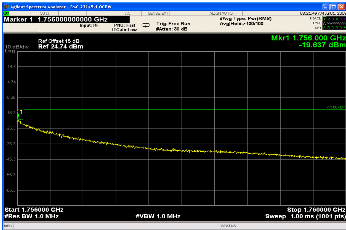
Channel 875 - Upper Band Edge
