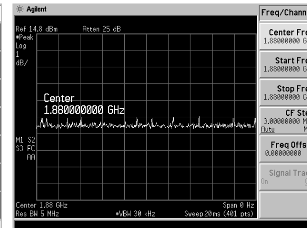
WCDMA 1880 MHz
