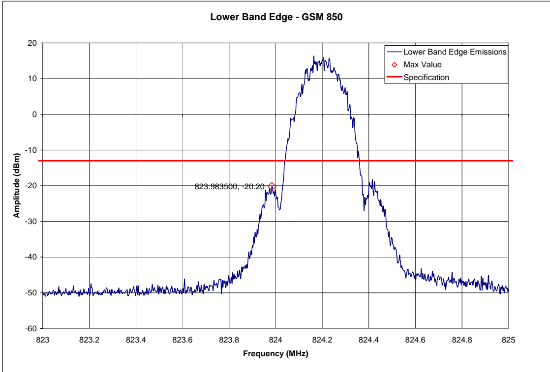
GSM 850 EDGE – Lower Band Edge – Channel 128 (824.2MHz)
