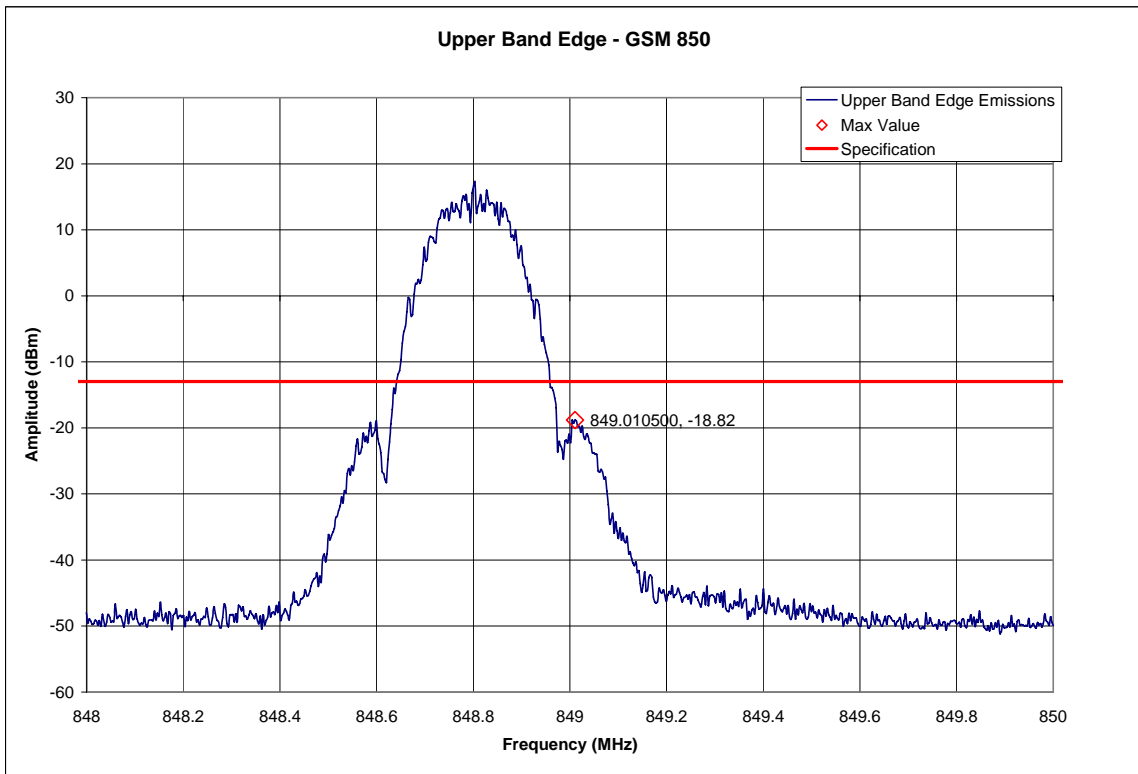
GSM 850 EDGE – Upper Band Edge – Channel 251 (848.8MHz)
