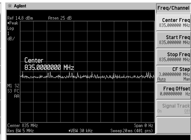
WCDMA 835 MHz
