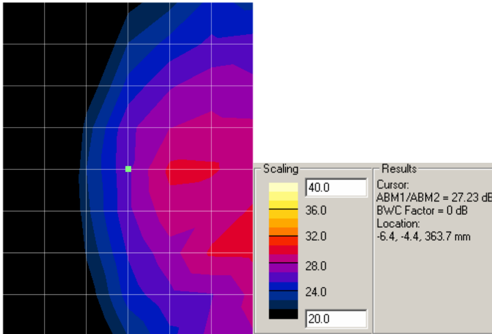
Radial1 – SNR
