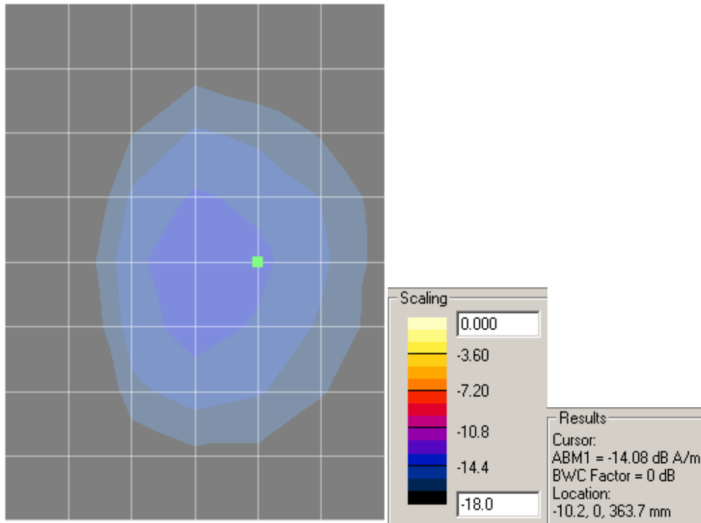
Radial1 – ABM1
