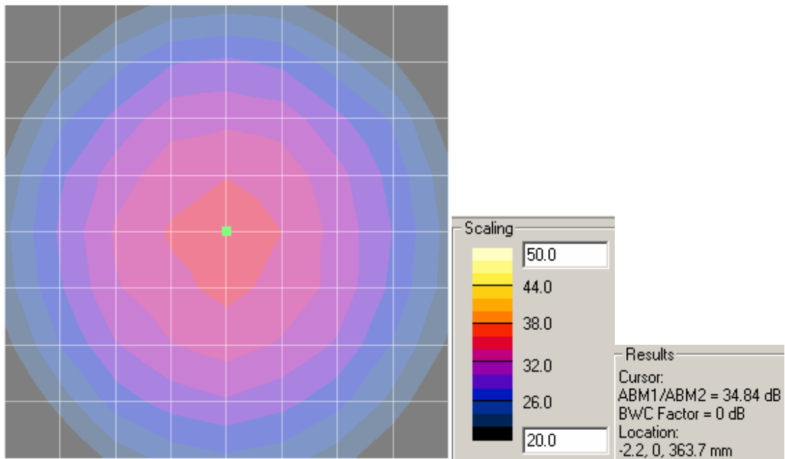
Axial – SNR
