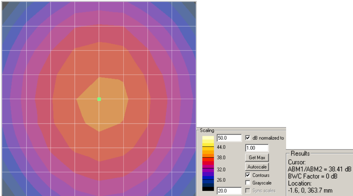
Axial - SNR
