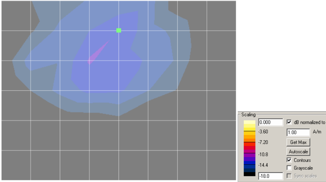
Radial2 - ABM1
