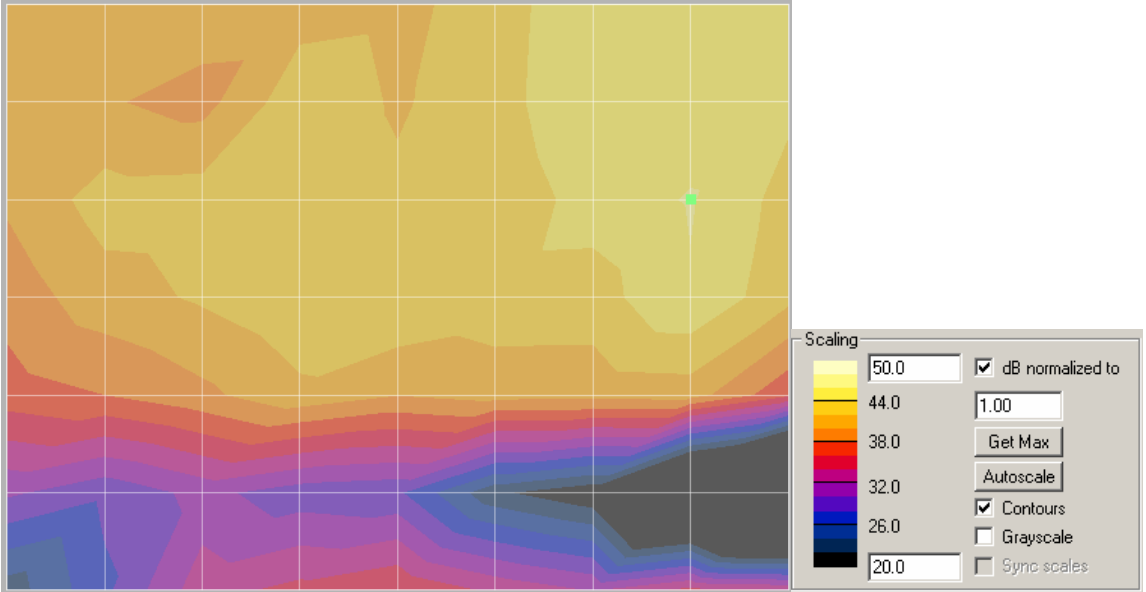
Radial 2 - SNR
