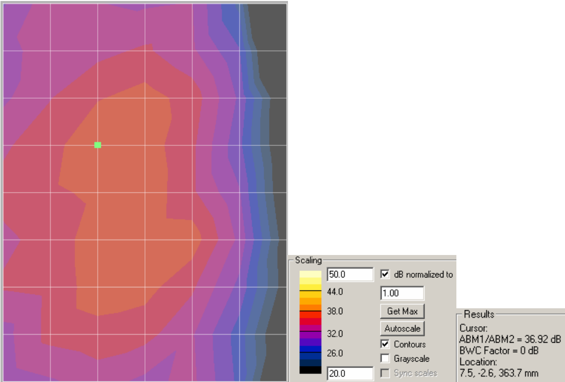
Radial 1 - SNR
