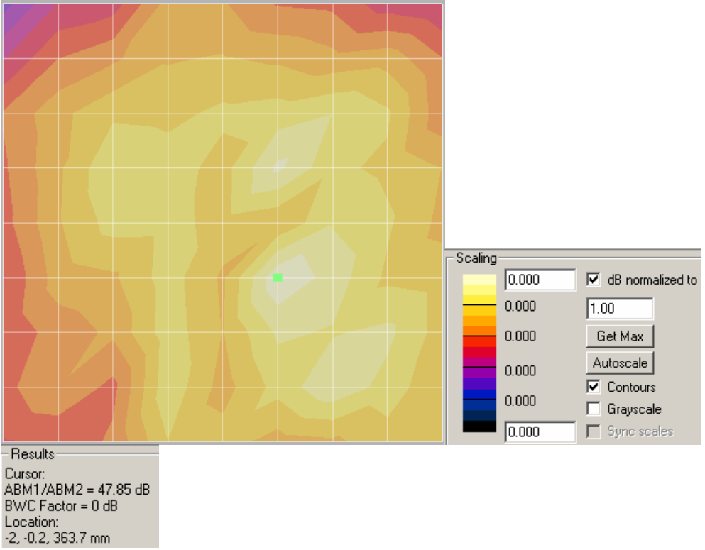
Axial - SNR
