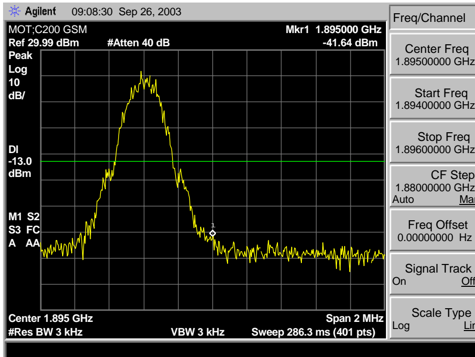
GSM 1900 Upper Band Edge
