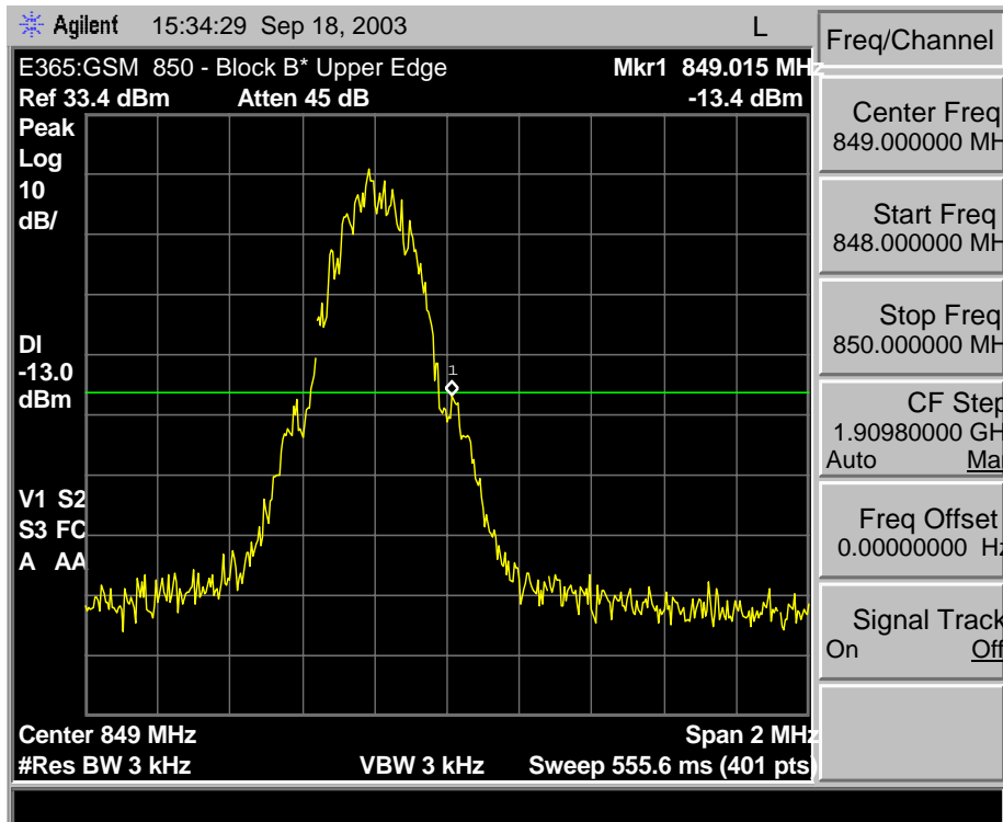
GSM 850 Upper Band Edge
