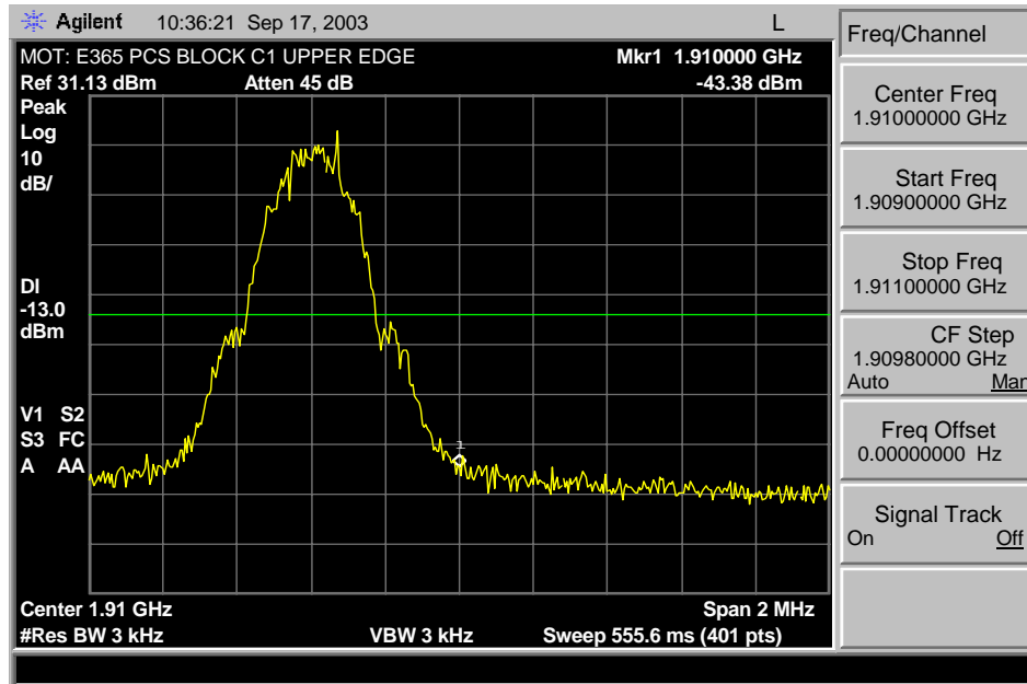
GSM 1900 Upper Band Edge
