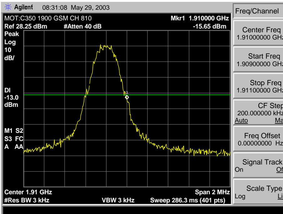
1900 GSM Upper Band Edge
