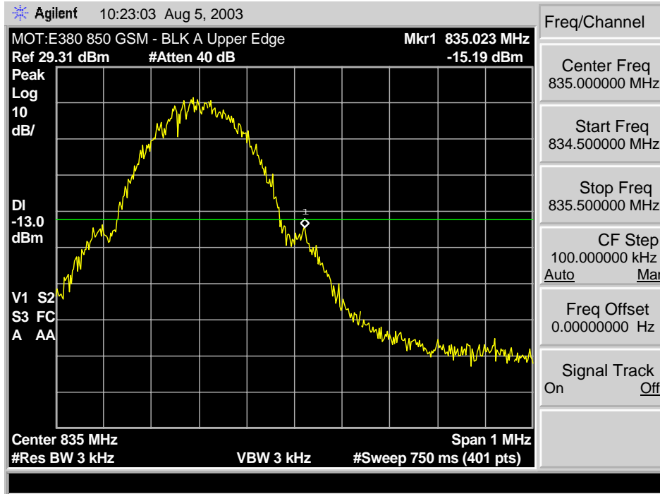
GSM 850 A Max/B Min. Block Edge
