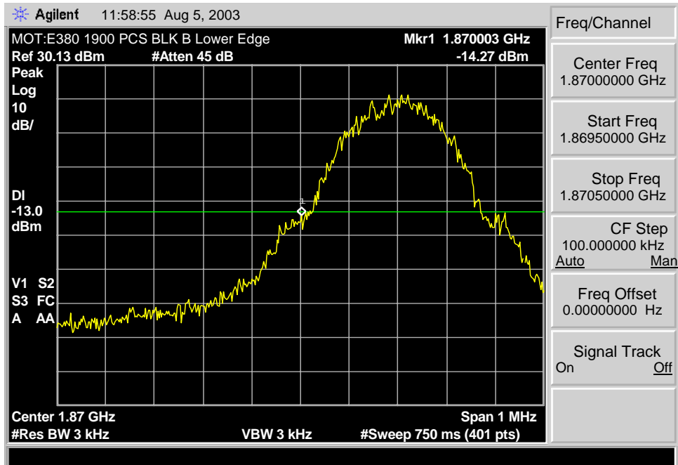
GSM 1900 B Min Block Edge
