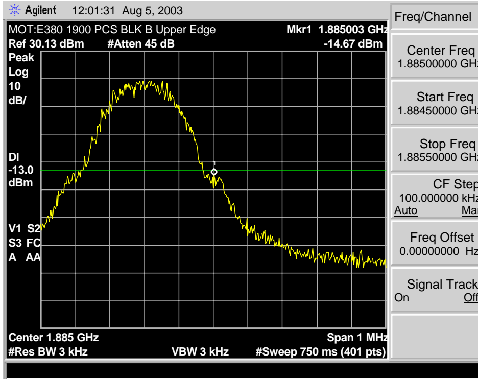
GSM 1900 B Max Block Edge
