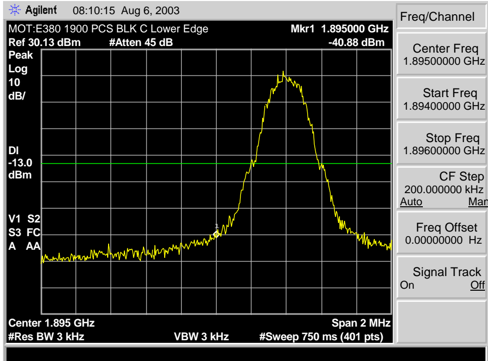
GSM 1900 C Min. Block Edge
