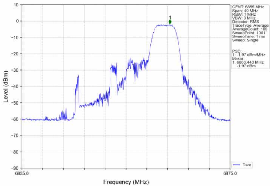
802.11ax(HEW20)_HCH_6855MHz_RU52_/_Ant4_NTNV
