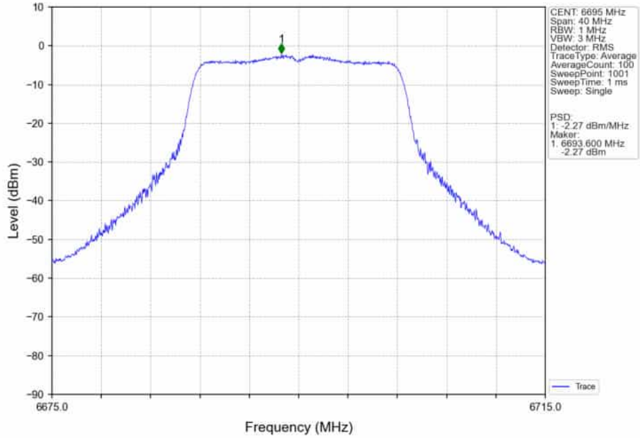
802.11a_MCH_6695MHz_MIMO_NTNV
