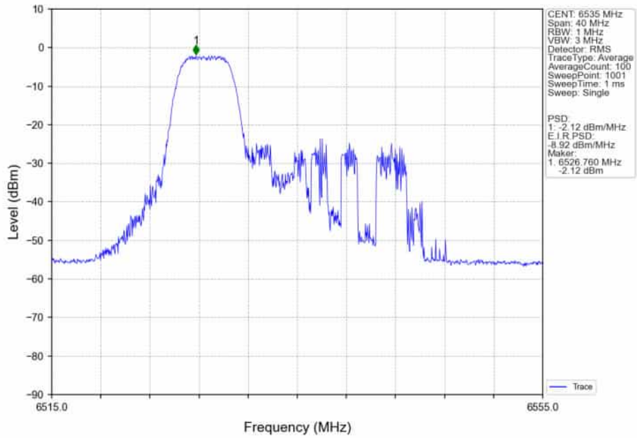
802.11ax(HEW20)_LCH_6535MHz_RU52_/_Ant4_NTNV
