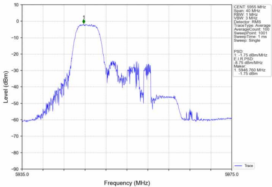
802.11ax(HEW20)_LCH_5955MHz_RU52/_Ant4_NTNV
