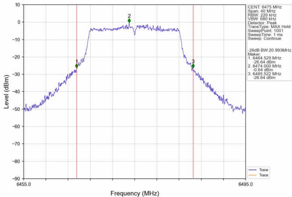
802.11a_MCH_6475MHz_Ant4_NTNV
