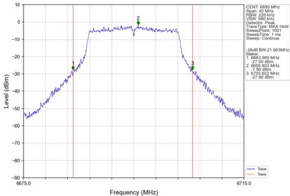
802.11a_MCH_6695MHz_Ant4_NTNV
