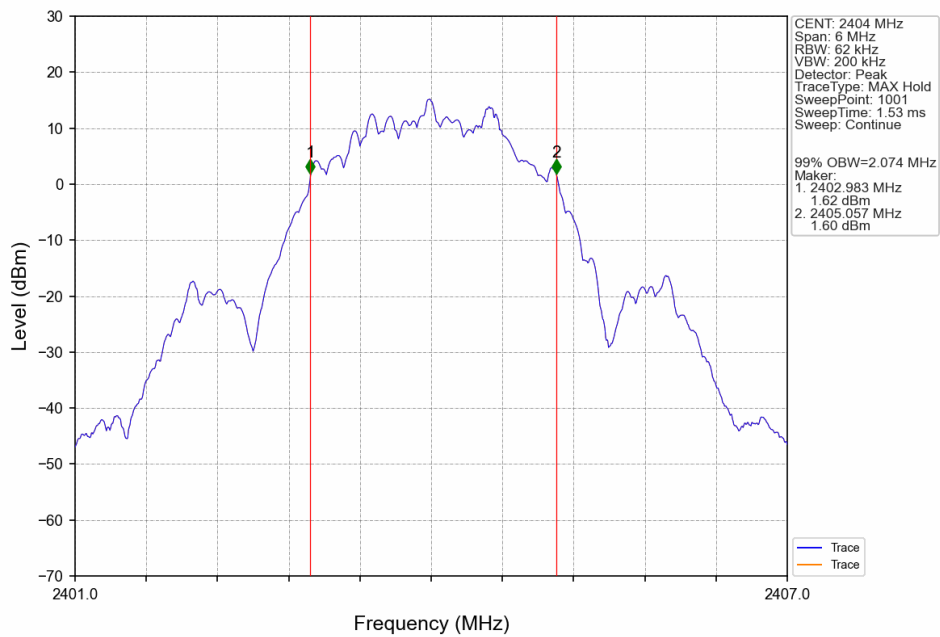
2M_LCH_2404MHz_Ant6_NTNV
