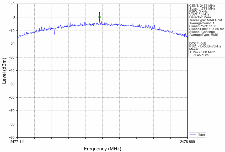
2M_HCH_2478MHz_Ant6_NTNV
