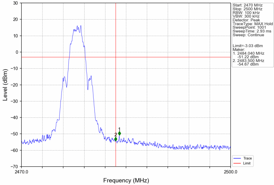
2M_HCH_2478MHz_Ant6_NTNV
