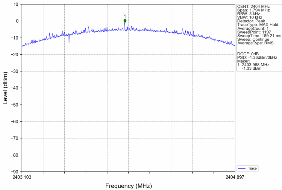
2M_LCH_2404MHz_Ant6_NTNV
