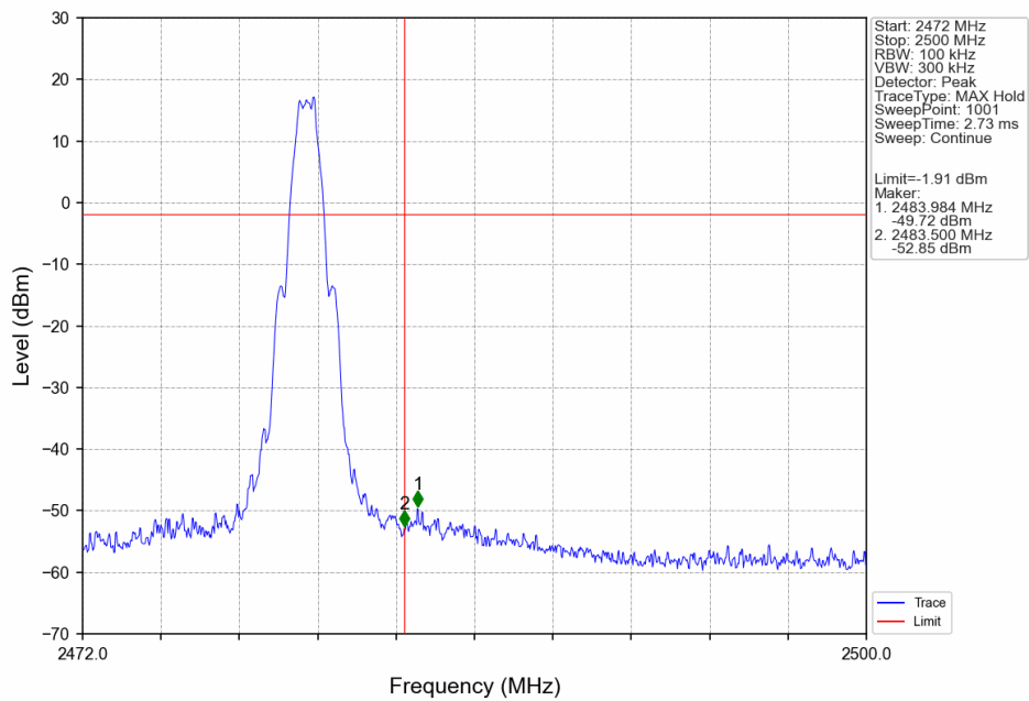
1M_HCH_2480MHz_Ant6_NTNV
