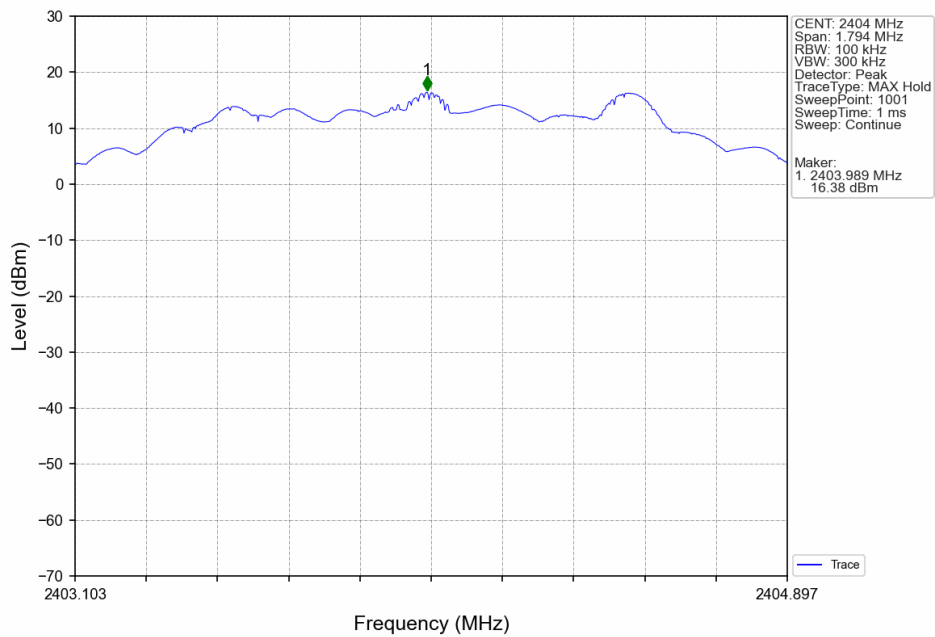
2M_LCH_2404MHz_Ant6_NTNV
