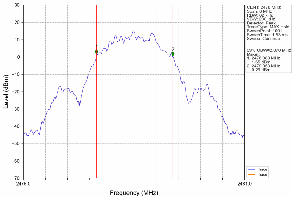
2M_HCH_2478MHz_Ant6_NTNV
