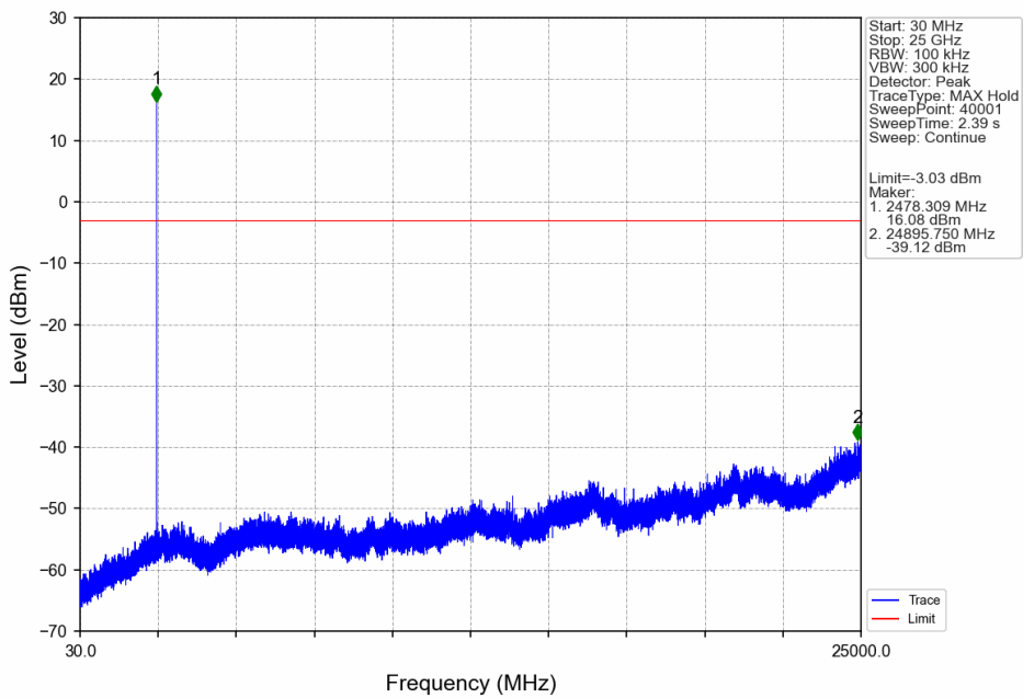
2M_HCH_2478MHz_Ant6_NTNV
