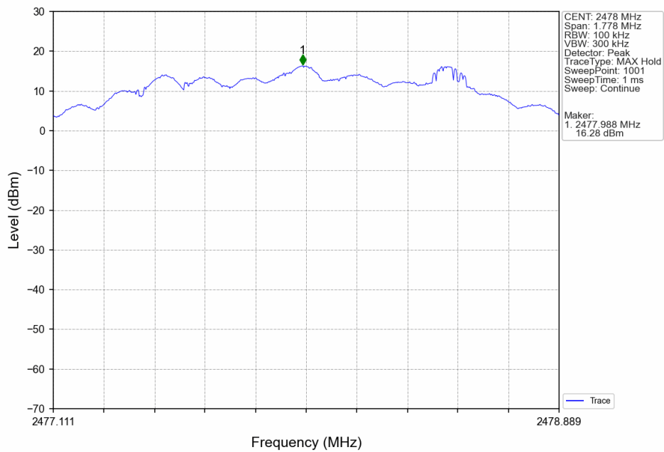
2M_HCH_2478MHz_Ant6_NTNV
