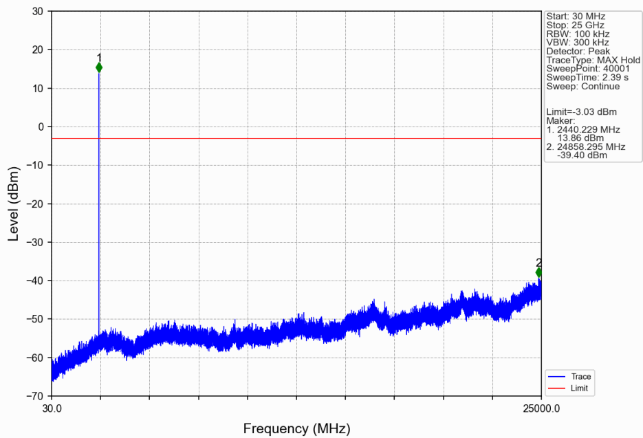
2M_MCH_2440MHz_Ant6_NTNV
