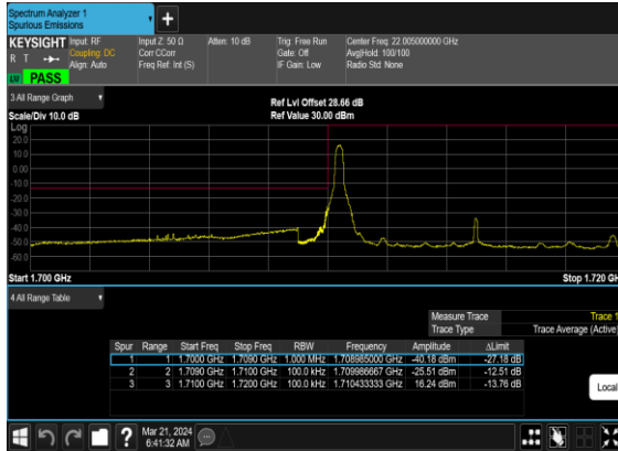
N66(10M)_CP- OFDM_QPSK_Edge_1RB_Left_Low_CH
