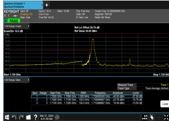
N66(10M)_CP-OFDM_16 QAM_Edge_1RB_Left_Low_CH
