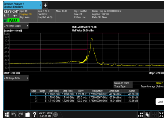
N66(25M)_CP-OFDM_16 QAM_Edge_1RB_Left_Low_CH
