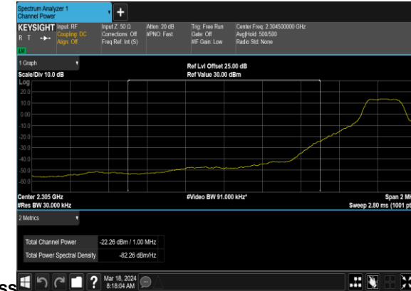
N30(5M)_DFT-s-OFDM_QPSK_Edge_1RB_Left_Low_CH_CHP_PA
