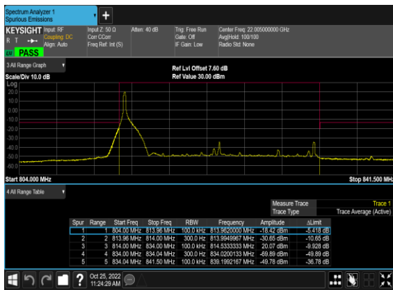
N26(20M)_DFT-s-OFDM_BPSK_Edge_1RB_Left_L ow_CH
