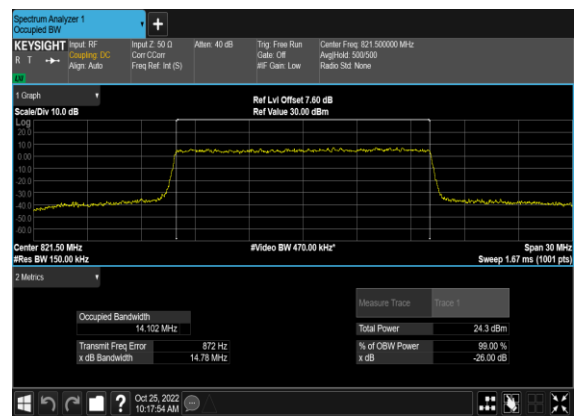
N26(15M)_CP-OFDM_256
