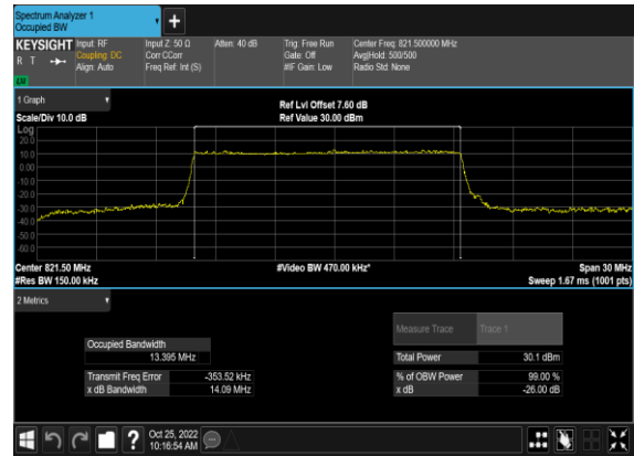
N26(15M)_CP-OFDM_16
