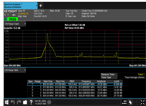
N26(20M)_DFT-s-OFDM_QPSK_Edge_1RB_Left_L ow_CH
