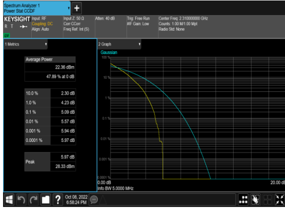
N30(5M)_DFT-s-OFDM_PI_2-BPSK_Outer_Full_
