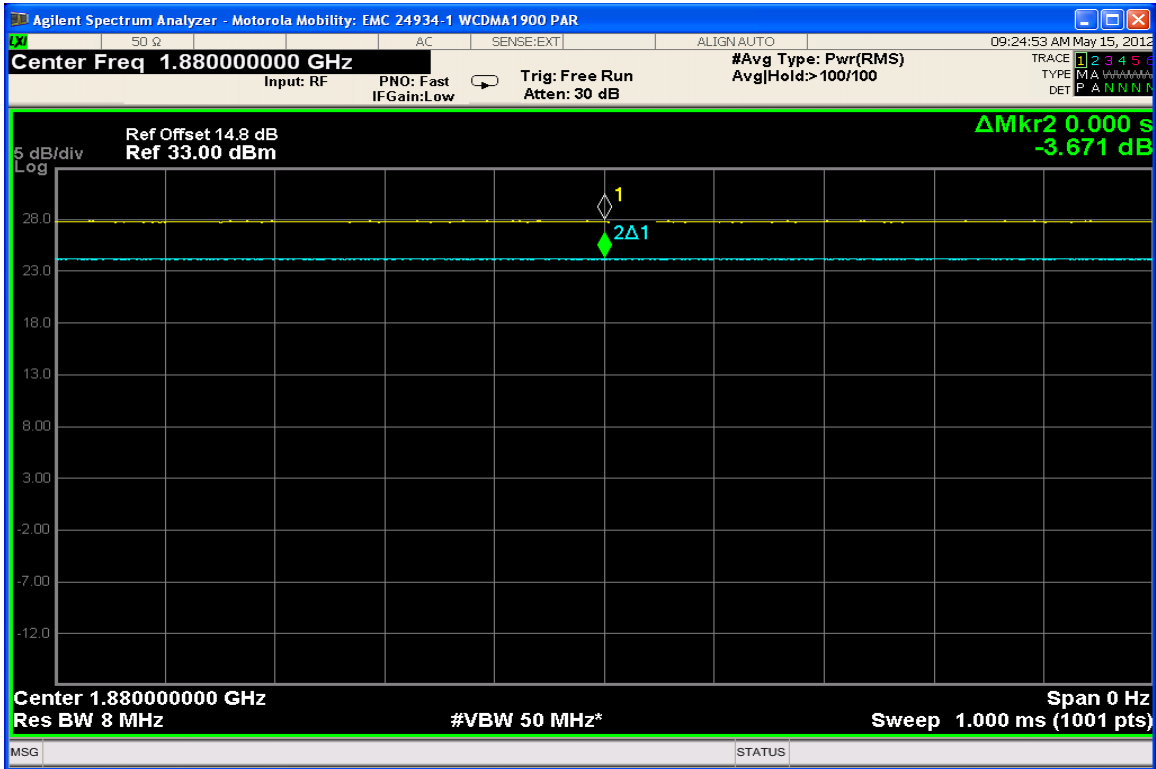
WCDMA 1900 – PAR Plot
