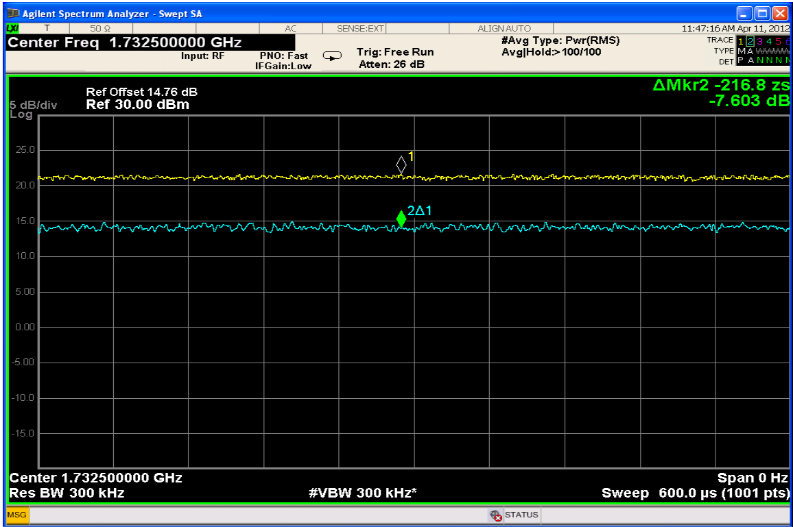
WCDMA 1700 – PAR Plot
