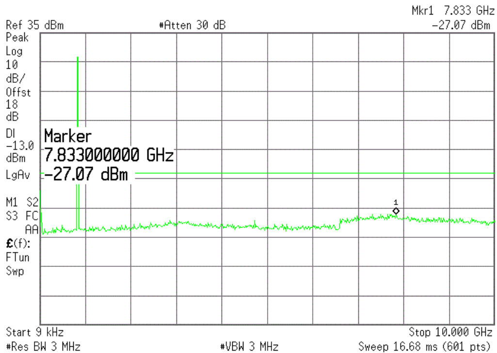
(Plot O4.:EGPRS 850MHz Channel = 251, 9KHz to 10GHz)
