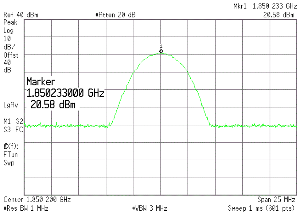
(Plot D6.2:EGPRS 1900MHz Channel = 512)
