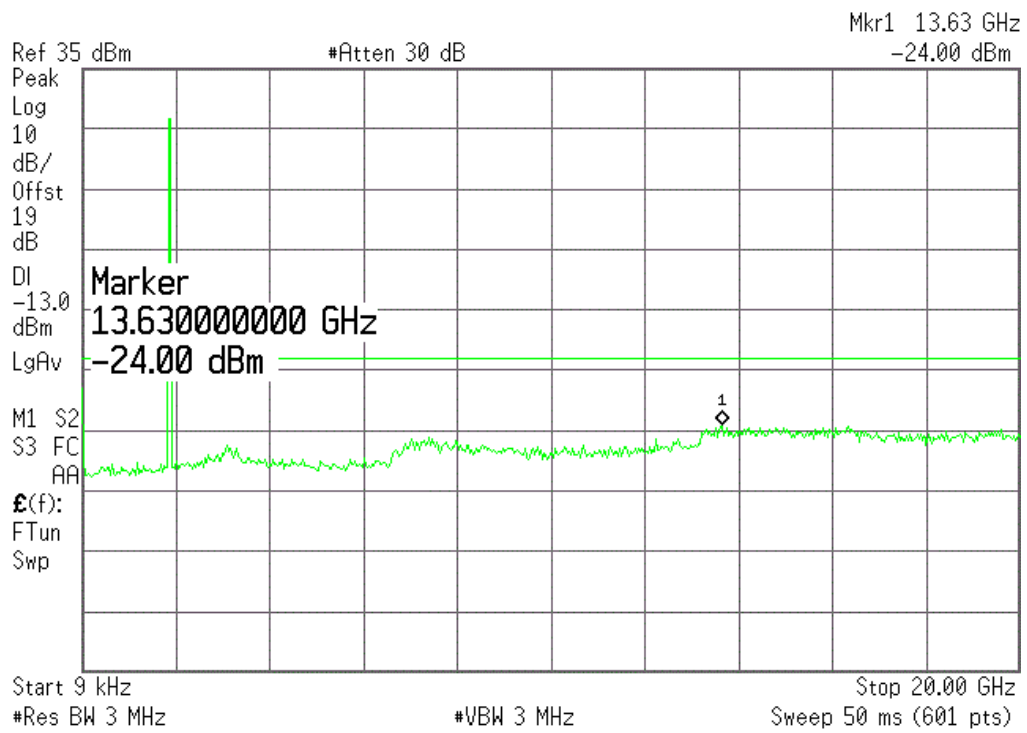
(Plot R4.:EGPRS 1900MHz Channel = 810, 9KHz to 20GHz)
