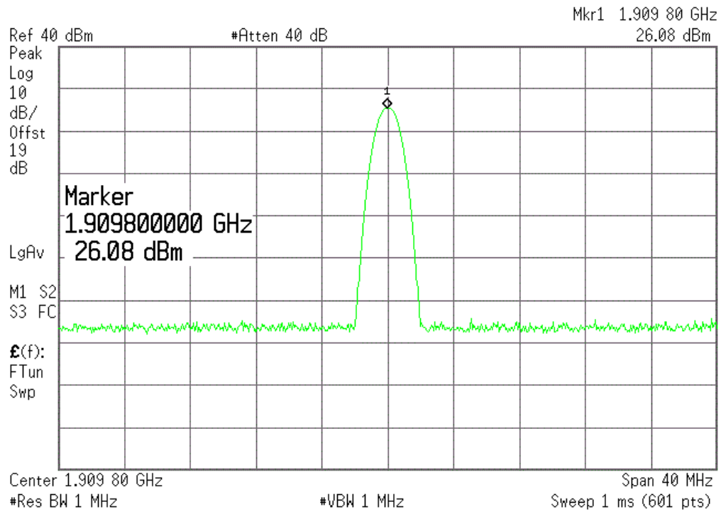
(Plot R2:EGPRS 1900MHz Channel = 810)
