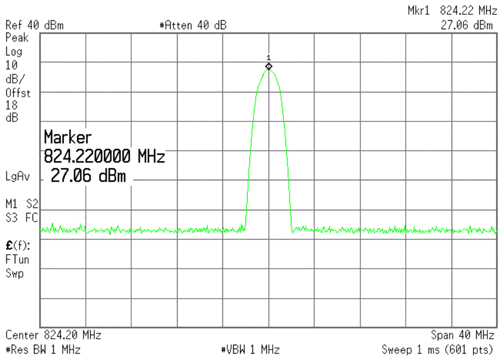
(Plot M2:EGPRS 850MHz Channel = 128)
