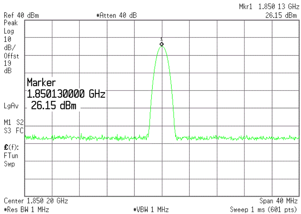
(Plot P2:EGPRS 1900MHz Channel = 512)
