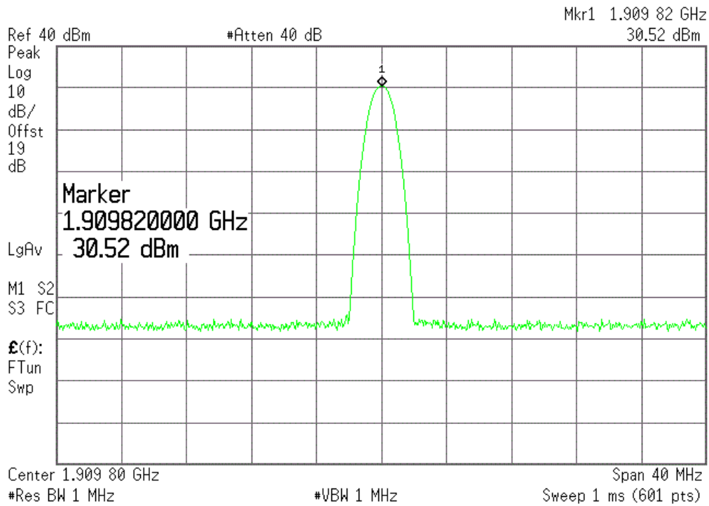
(Plot F2: GSM 1900MHz Channel = 810)
