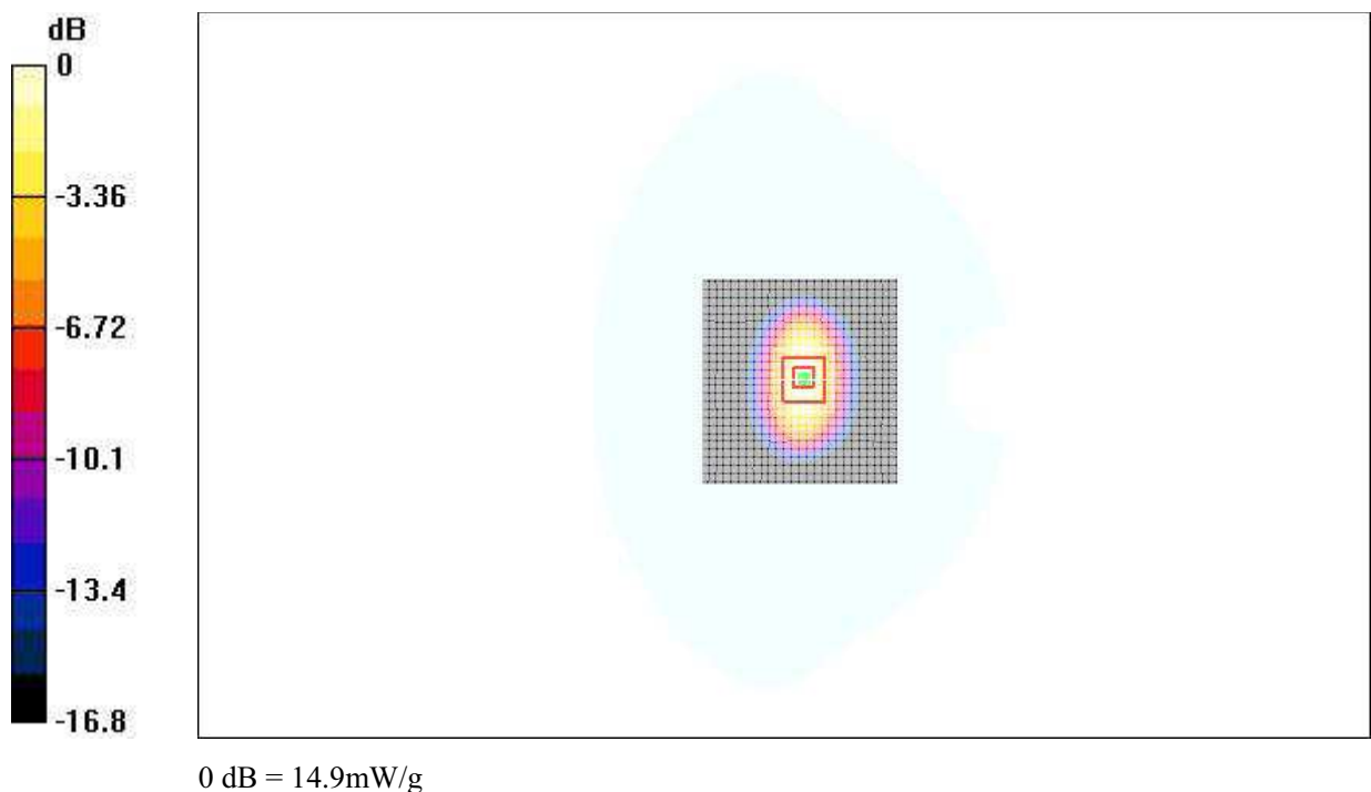
Fig.37 validation 2450MHz 250mW
