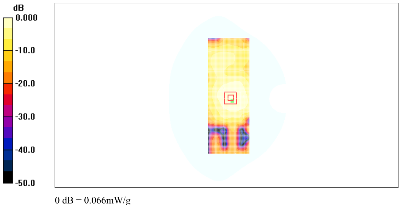
Fig. 31 2450MHz CH1
