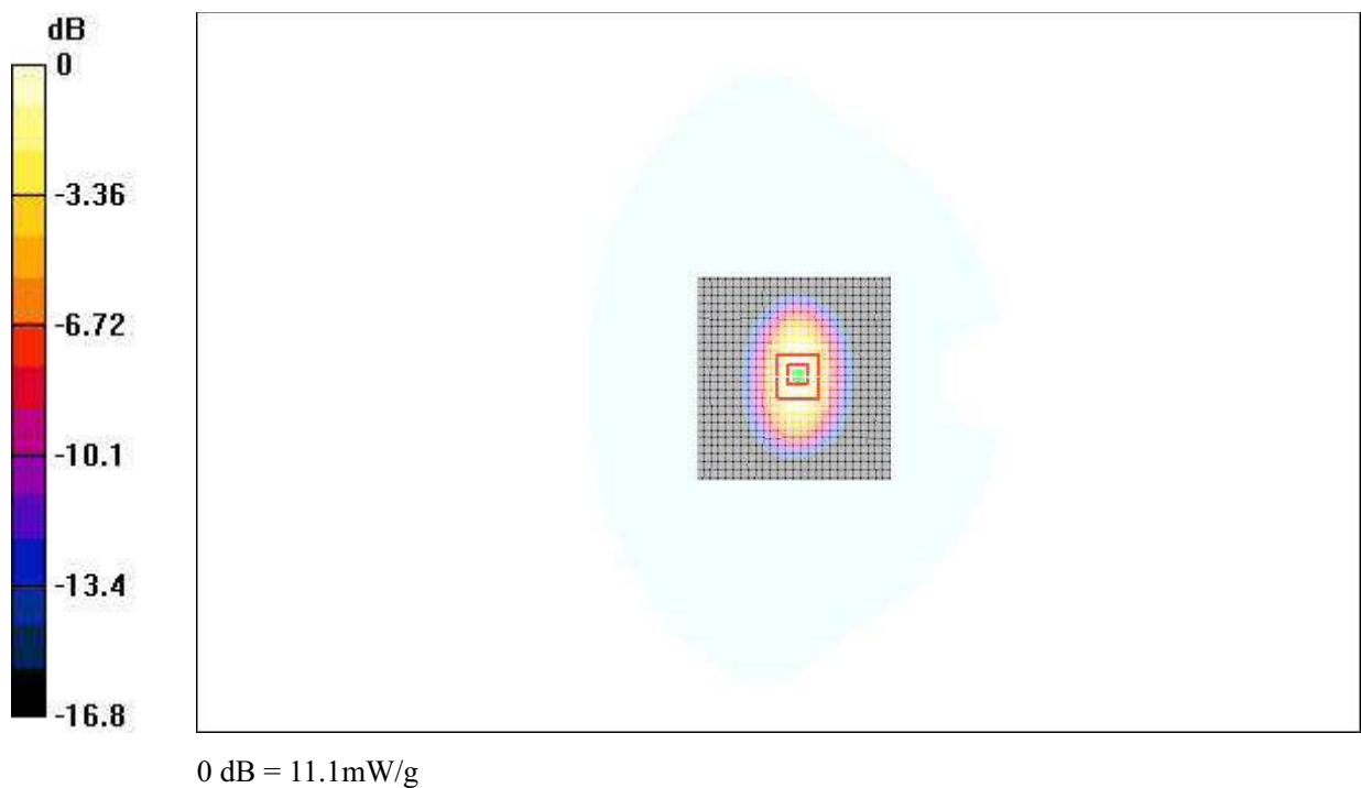
Fig.35 validation 1900MHz 250mW
