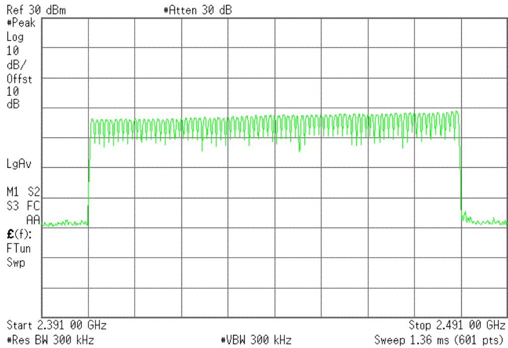
(Plot A: 2402MHz to 2480MHz)
