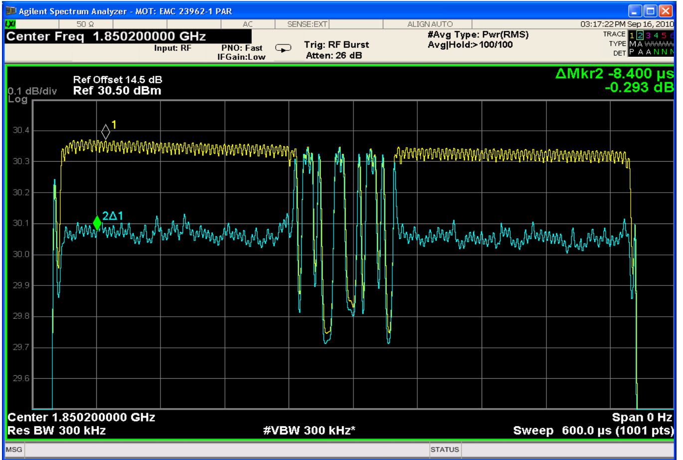
GSM 1900 – PAR Plot
