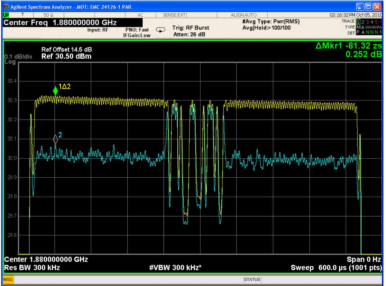
GSM 1900 – PAR Plot
