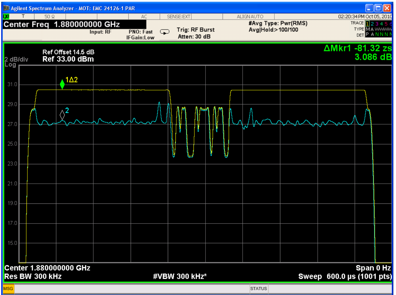
EDGE 1900 – PAR Plot
