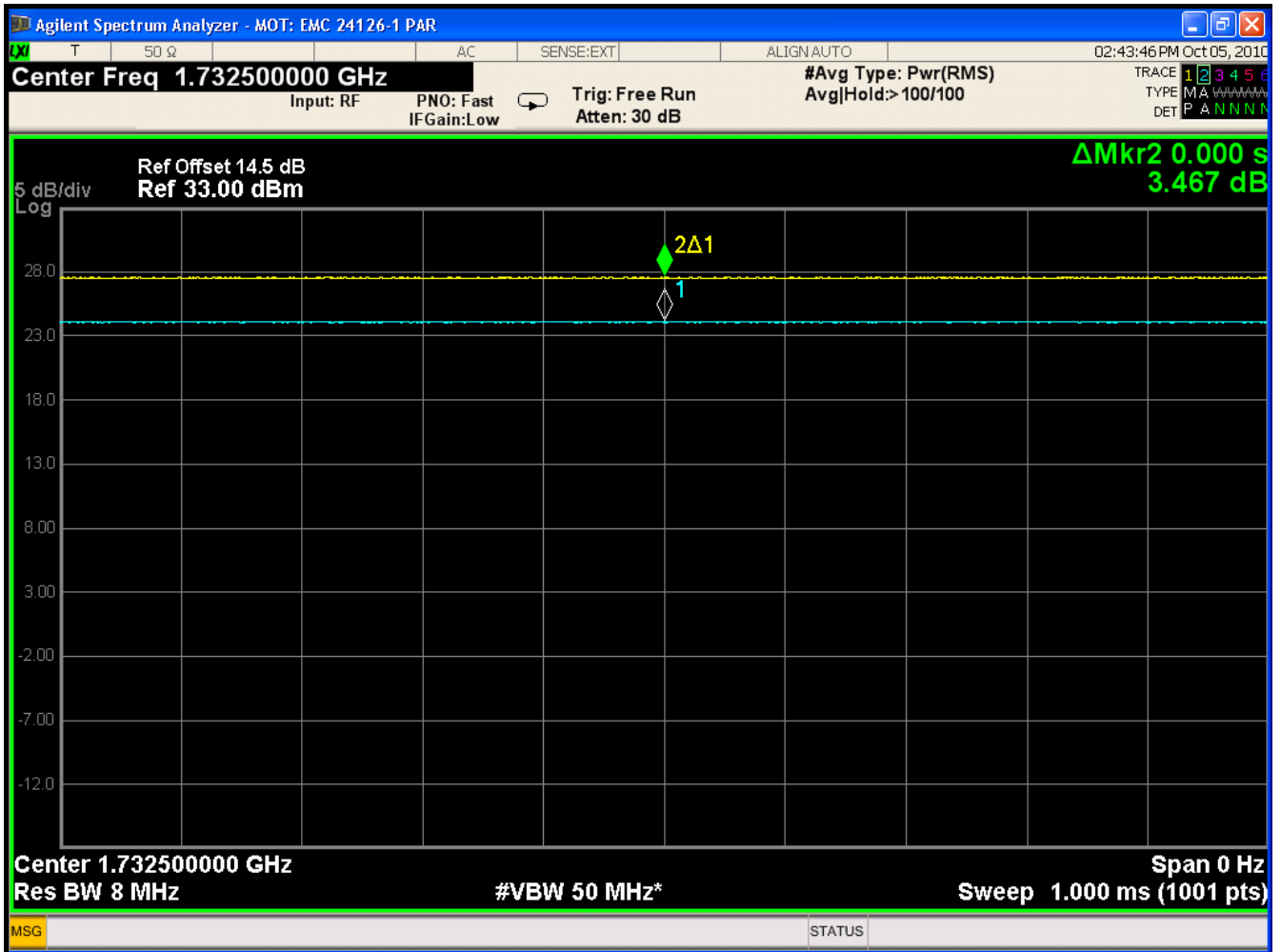
WCDMA 1700 – PAR Plot
