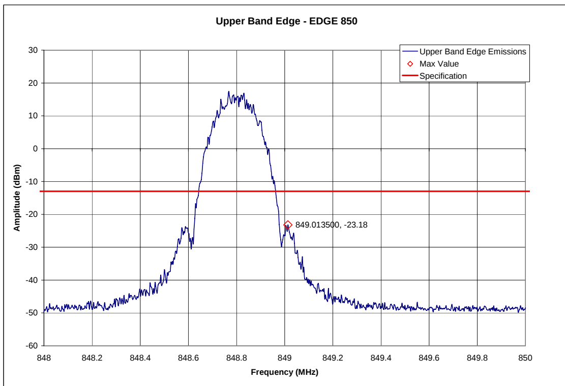
EDGE 850 – Upper Band Edge – Channel 251 (848.8 MHz)
