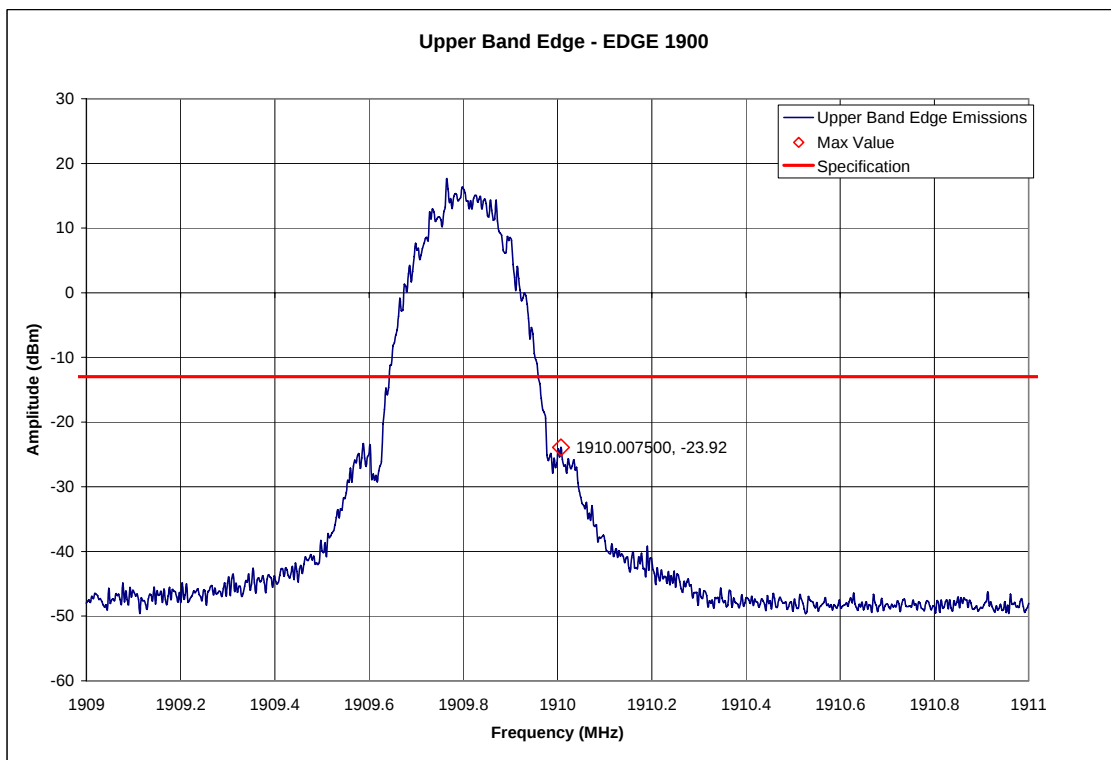
GSM 1900 EDGE – Upper Band Edge – Channel 810 (1909.8MHz)
