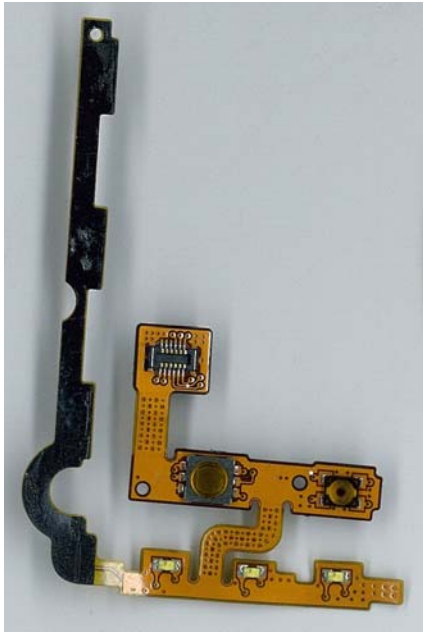
Bottom Key Flex Top
