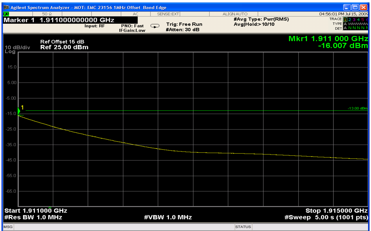
Channel 1175 Upper Band Edge
