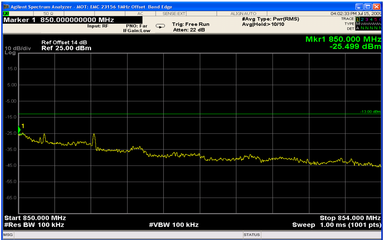
Channel 777 - Upper Band Edge
