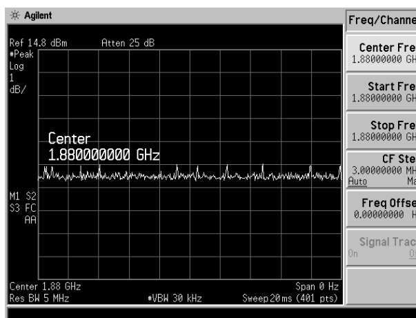
WCDMA 1880 MHz
