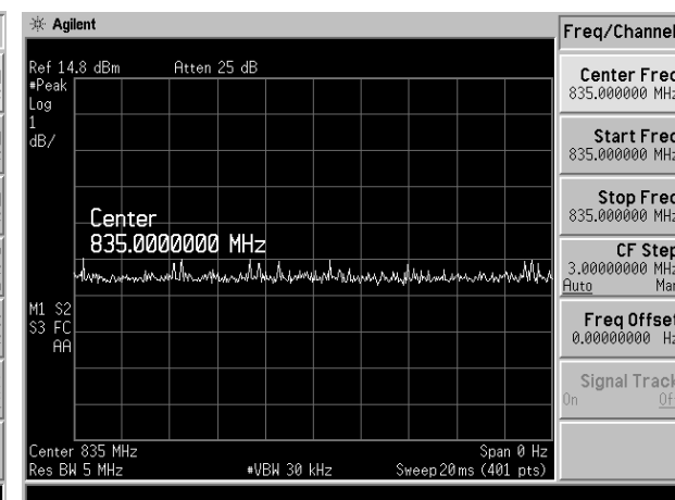
WCDMA 835 MHz
