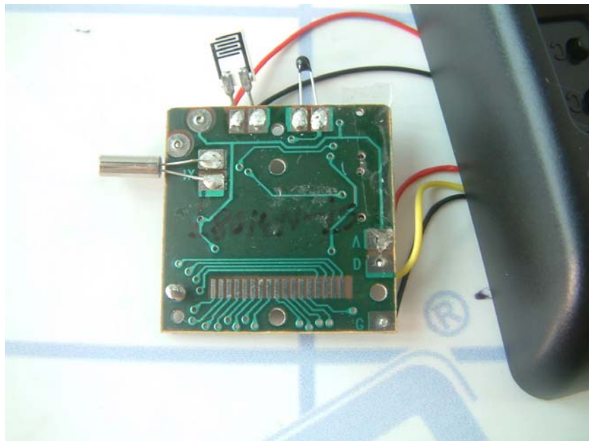
PCB 1 side2
