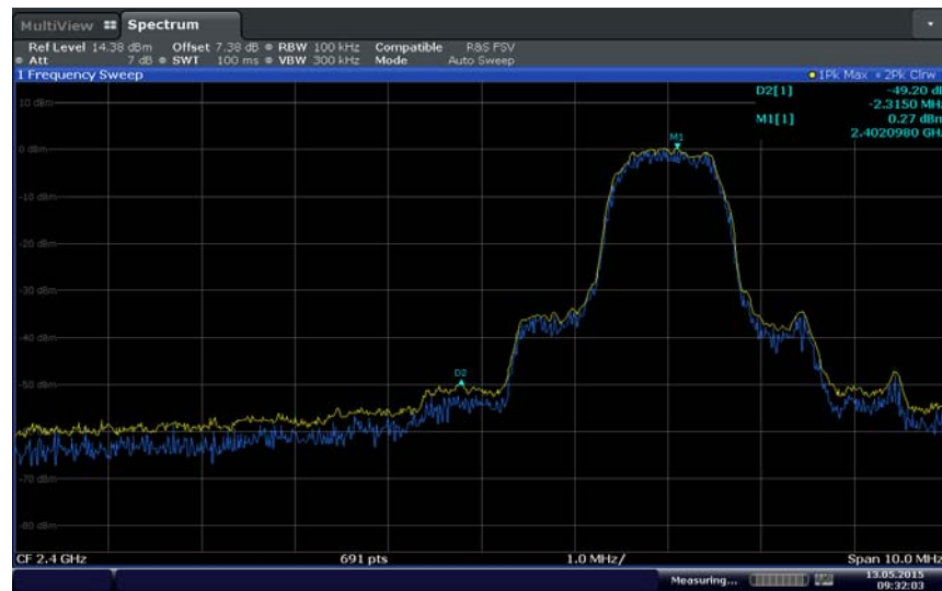
Non-hopping lower band edge (8DPSK)
