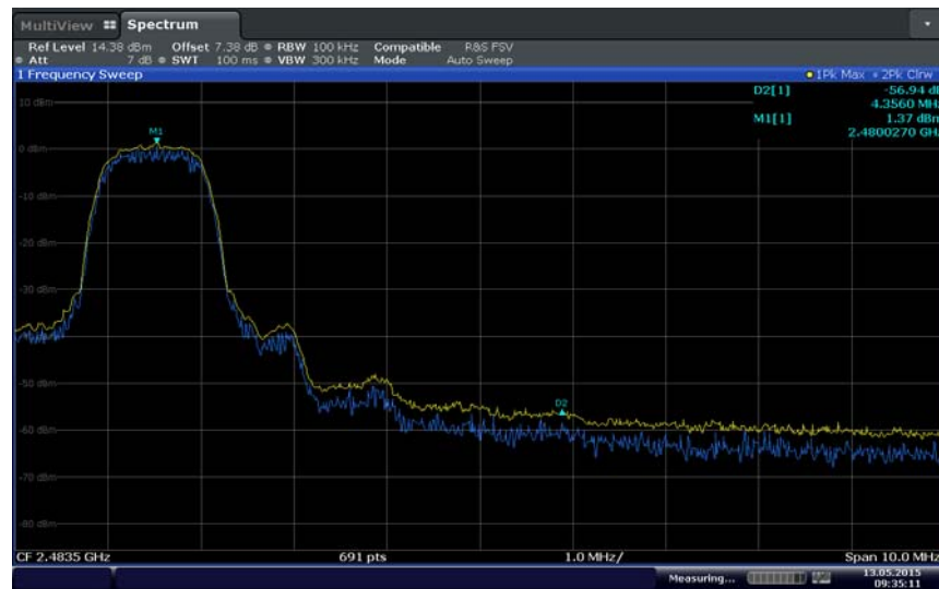
Non-hopping upper band edge ( \pi/4 -DQPSK)
