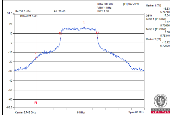
802.11a_Chain2 / CH149
