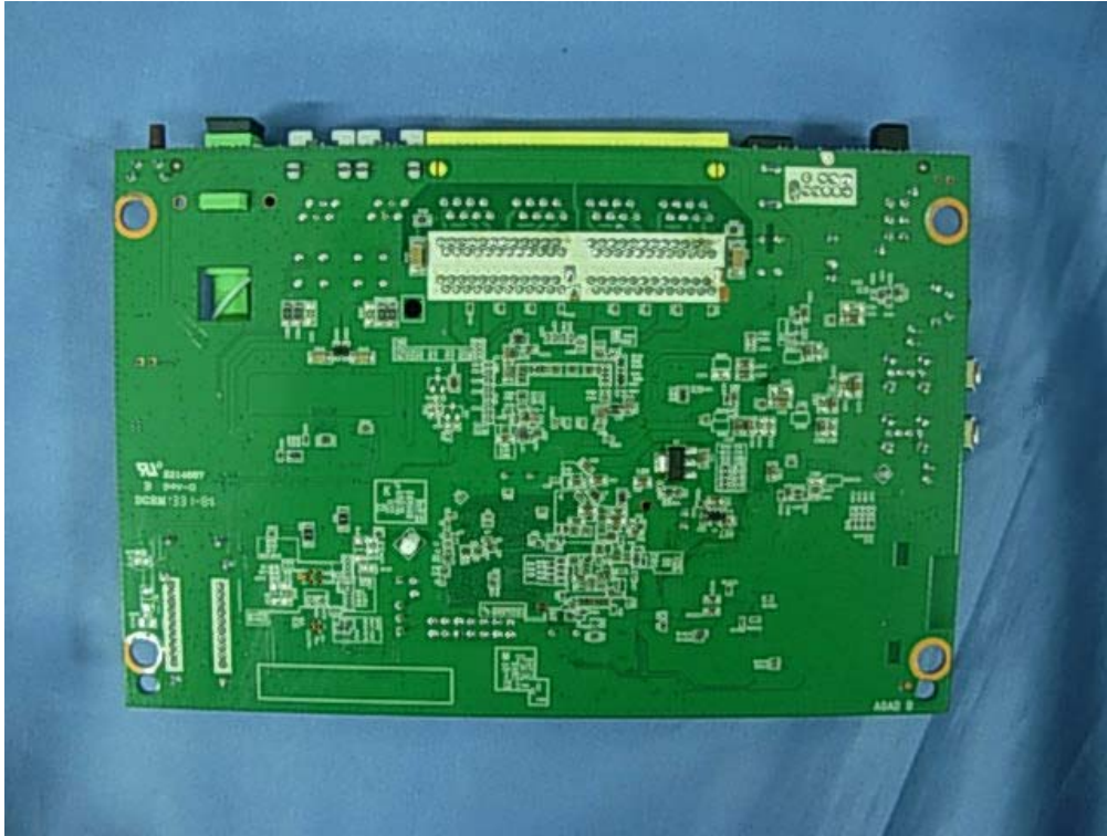
(16) EUT Photo
