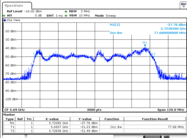
HE80 CH 138
