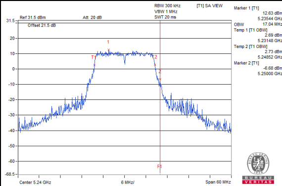
802.11a_Chain 2 / CH48
