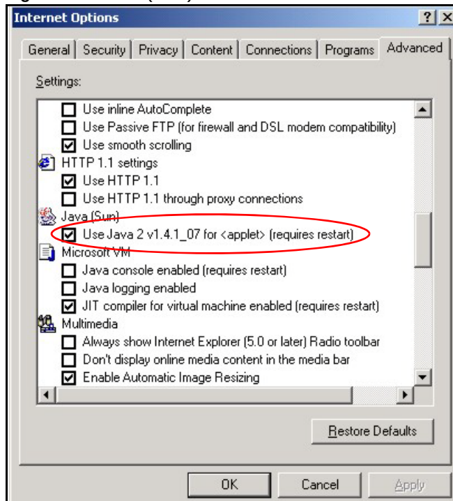
Figure 170 Java (Sun)
