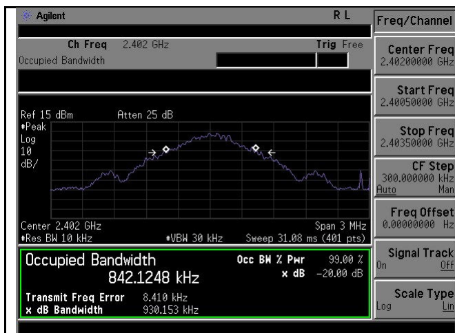
20dB Low CH 2402 - BDR
