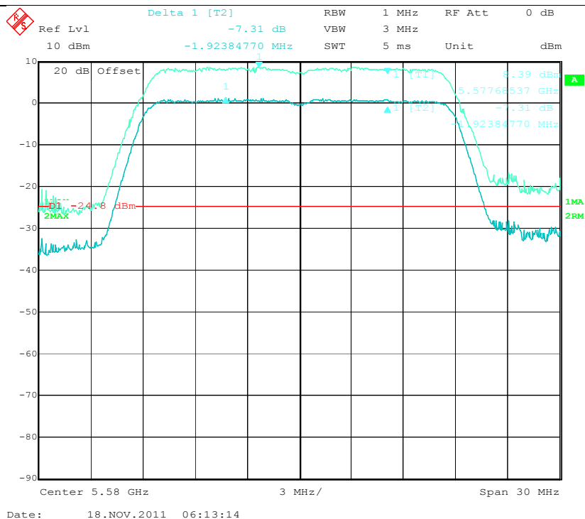
N-20MHz – 5.6GHz – Mid
