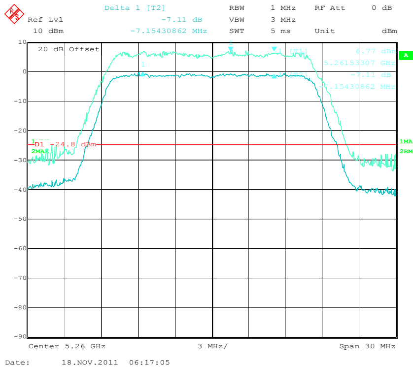
A-20MHz – 5.2GHz - Low
