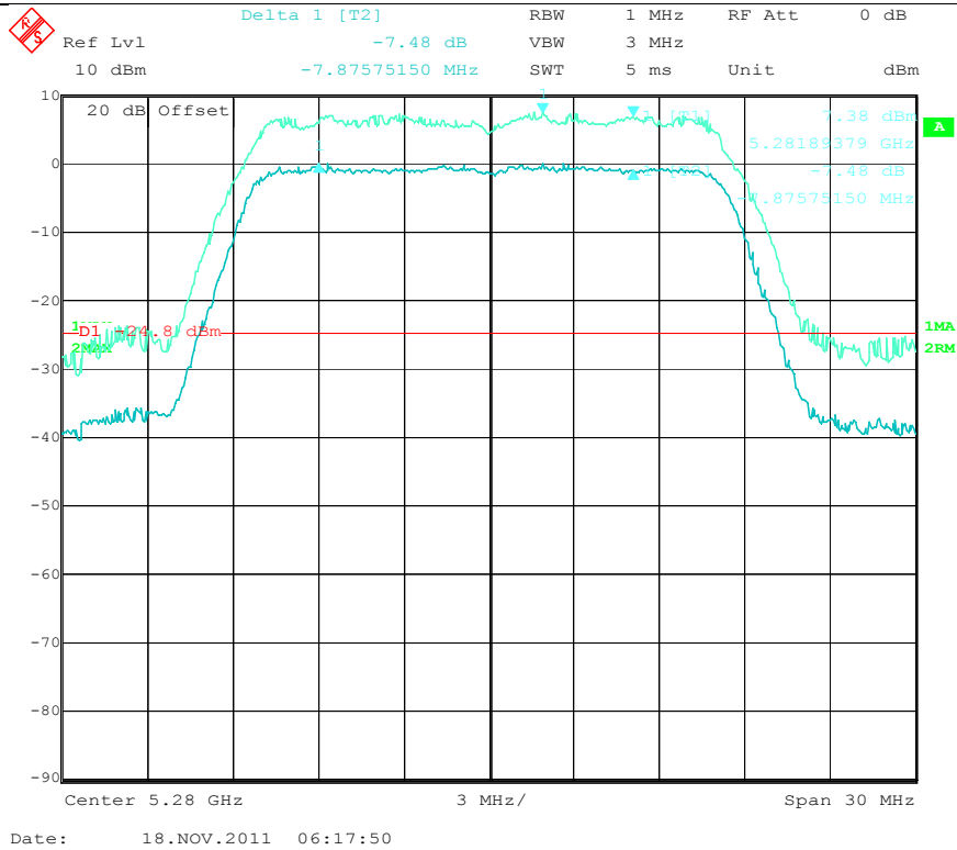
A-20MHz – 5.2GHz - Mid
