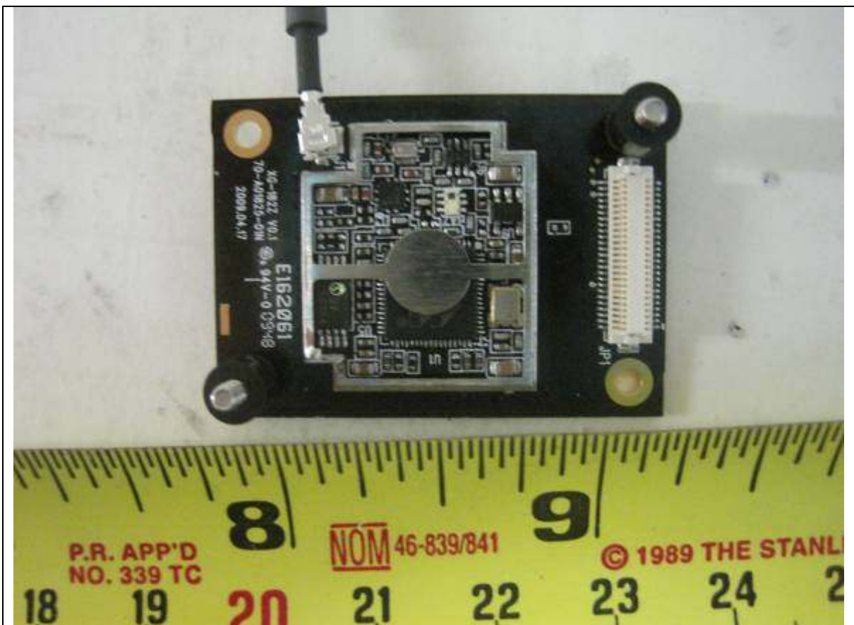
EUT : RF Module Component View
