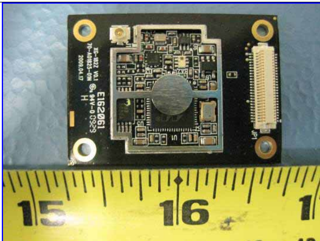
EUT : RF Module Component View
