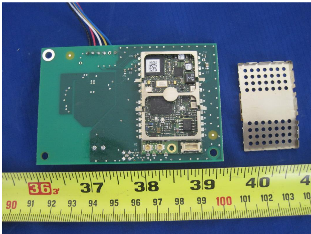
RFID Module-Bottom View
