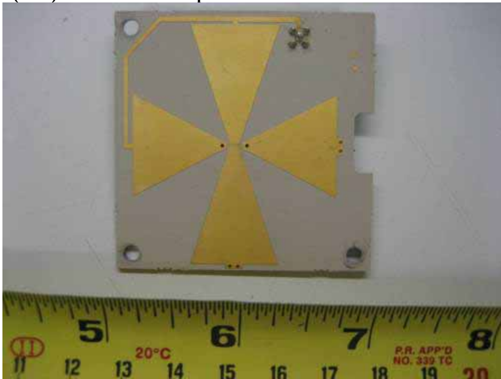
RFID (UHF) Module Antenna-Bottom
