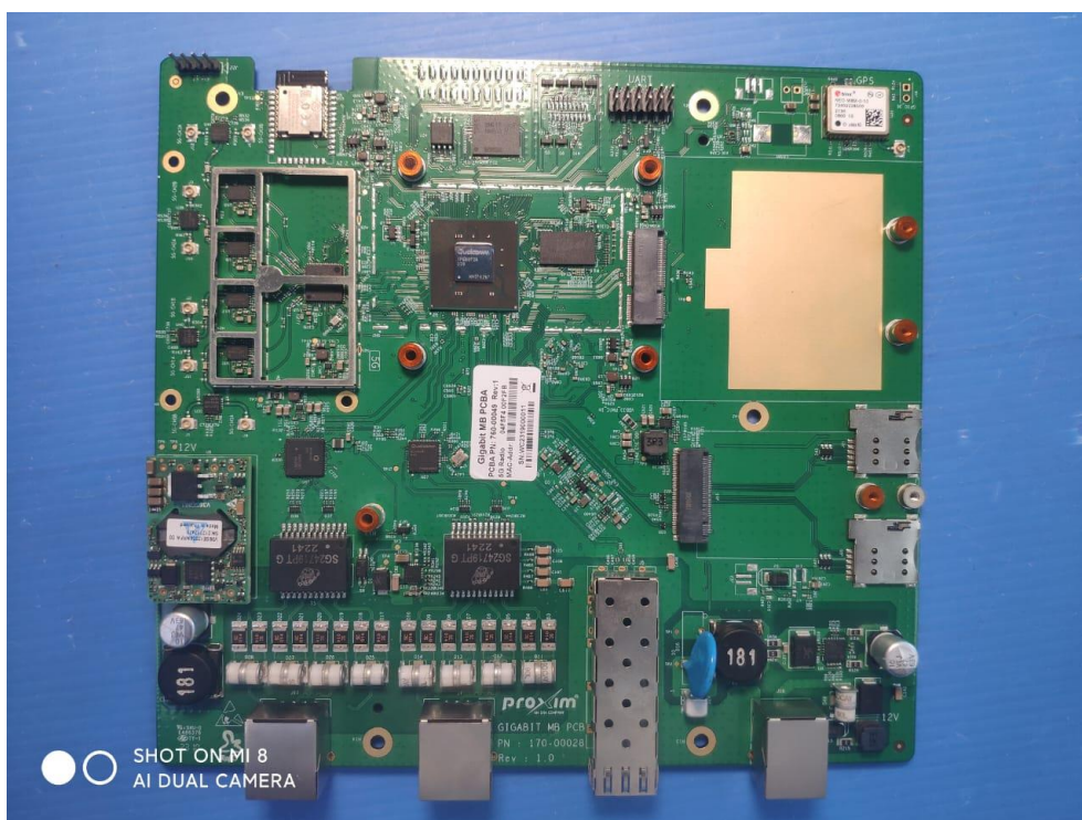
PCB Module without encloser
