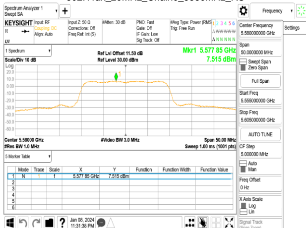
802.11ax_20MHz_Chain0_5580MHz_SU
