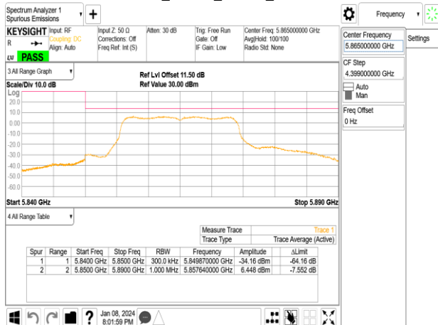
802.11n_20MHz_Chain0_5865MHz
