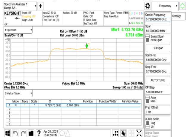
802.11ax_20MHz_Chain0_5720MHz_UNII 2C_SU
